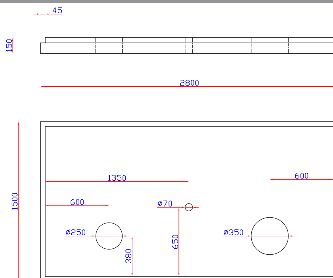
Betonplatform til råvandsstation Mega
