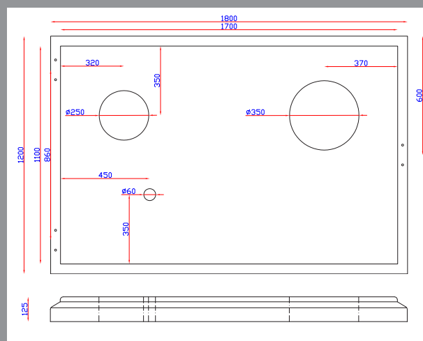
Betonplatform til råvandsstation Compact og Universal
